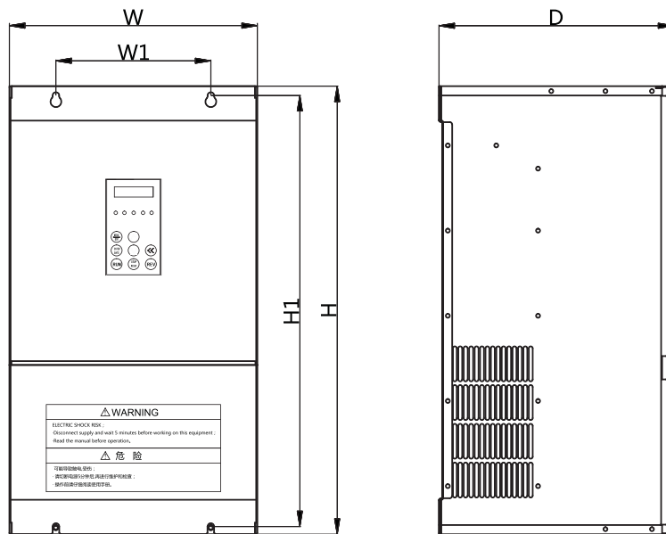
CV22 系列塔机回转专用变频器外形尺寸和安装尺寸一览表
